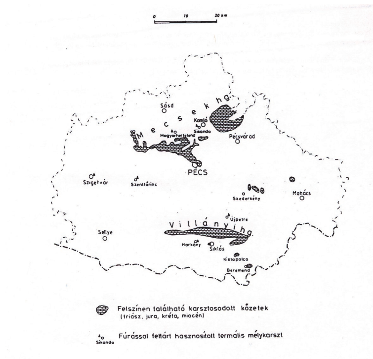
4. ábra. Karsztosodott képződmények elterjedése Baranya megyében. (Rónaki 1997. p.45.)
