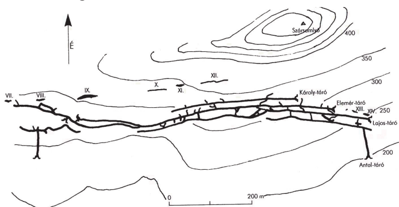
17. ábra. A szársomlyói (nagyharsányi) bauxitbánya térképe.
