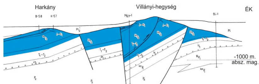
15. ábra. A villányi hegység legújabb földtani szelvénye.
