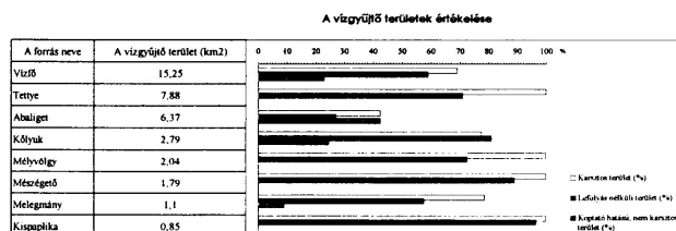
13. ábra. A nagy mecseki karsztforrások vízgyűjtő területei.
