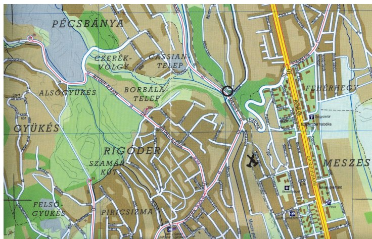
3. ábra. A pécsbányatelepi kiszáradt Sárkány-forrás és a hajdani Cassian-akna helye a mai 2003-as térképen általunk feltüntetve.
