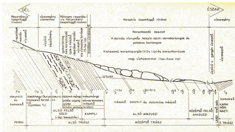
11. ábra. Idealizált földtani szelvény.
