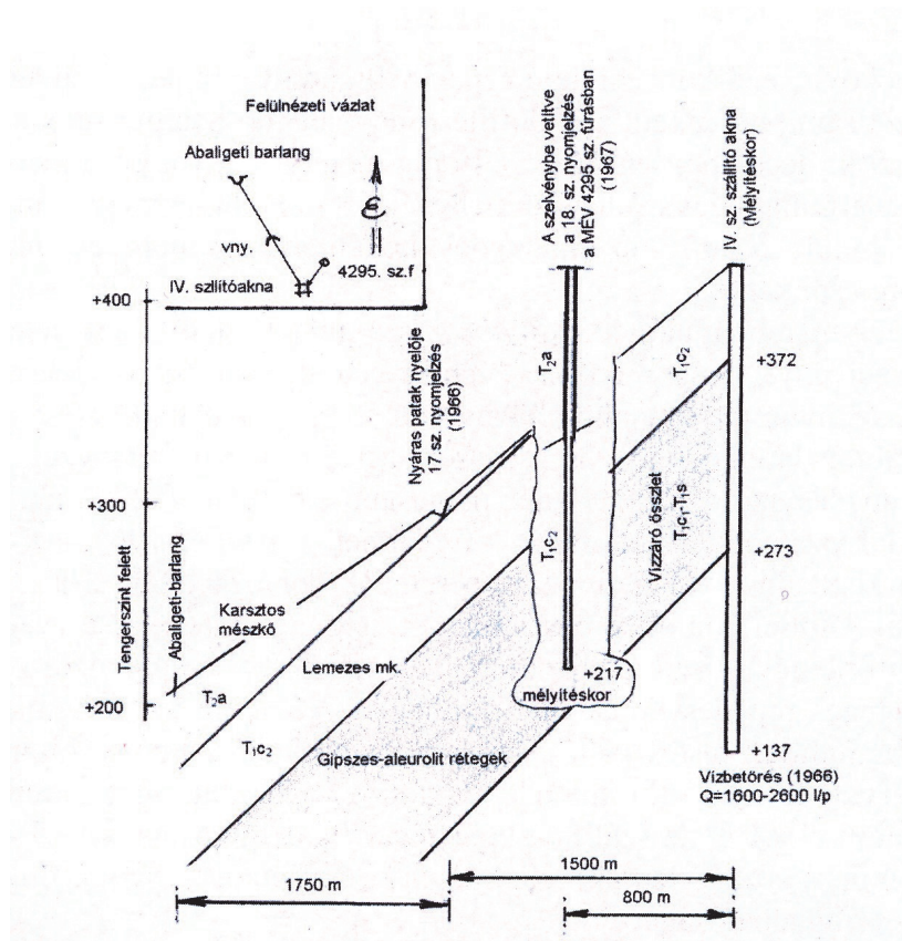
10. sz. ábra. Egy víznyomjelzés földtani környezete.
