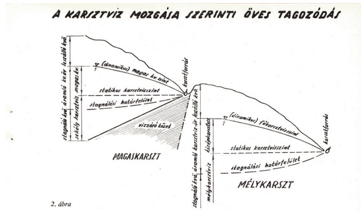
2. ábra. A karsztvíz mozgása szerinti öves tagozódás. (u.ott, p.79.)
