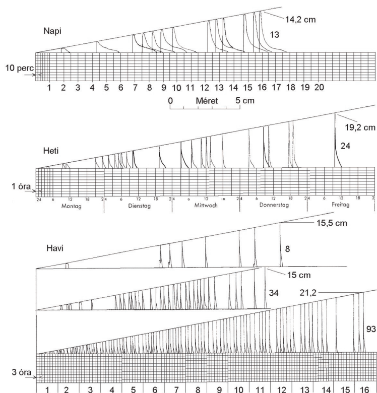
8. ábra. Különböző kitörési formák.
