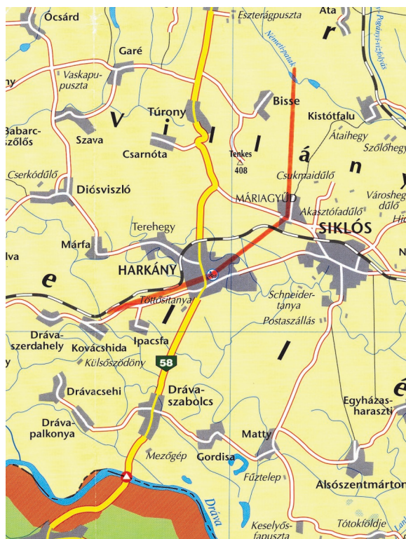
16. ábra. Térképrészlet a földtani szelvényvonallal.
