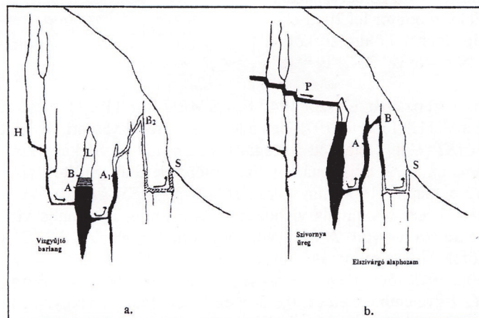
6. ábra. A Sárkány-kút szivornyájának elvi vázlata a régi (a) és az új (b) elképzelés szerint. a): H = vizgyűjtő réshálózat, L = légszák, B, A = vízszint kiömlés elején és végén, A 1 és B 1 közötti szakasz = vízszint-emelkedés változása kitörés előtt, b): P = patakmeder, A = leszívó cső, B = leszívó cső csúcspontja. Mindkét oldalon: S = a forrás helye.
