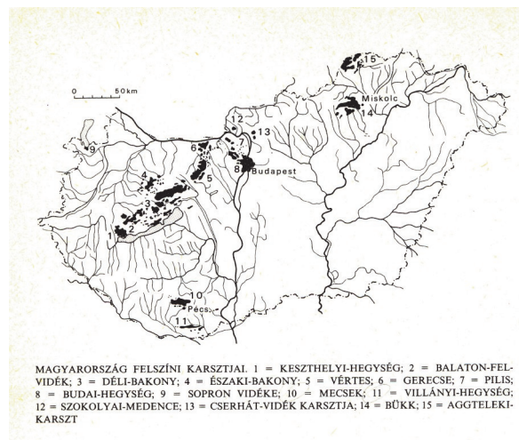
3. ábra. Magyarország felszíni karsztjai. (Kordos 1984. p.32.)
